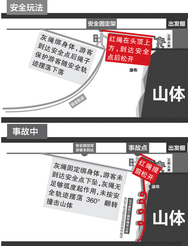
网友对“瀑布秋千”事故的分析图 图片来源于网络
