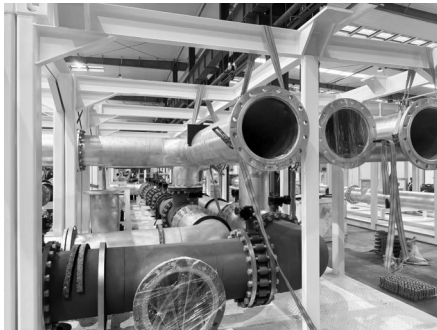
冷却方舱的管道
